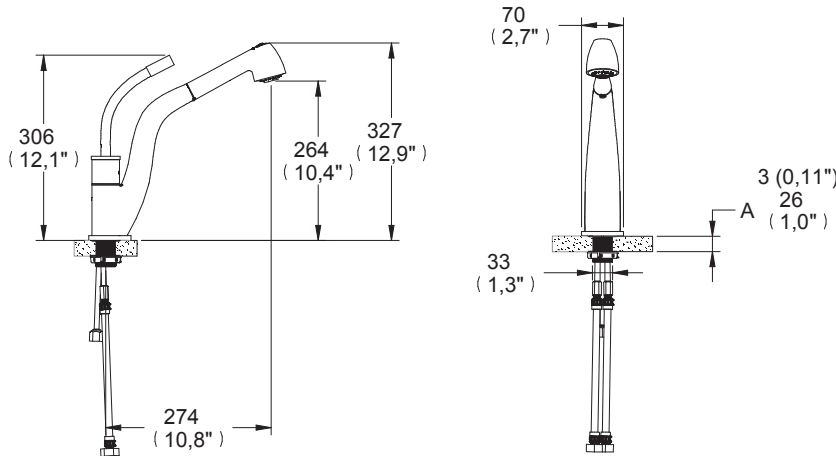
Medidas Referenciales / Estimated Dimensions, Acot.mm.(pulg) / Dim.mm.(in)
